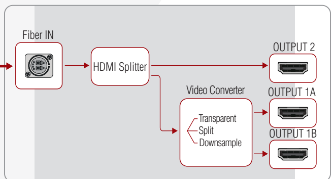
HDMI20-OPTC-RX220-Pro
