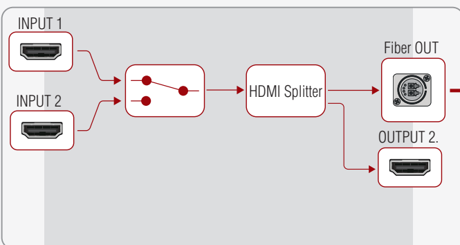
HDMI20-OPTC-TX220-Pro
